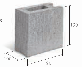
1/2隅形
